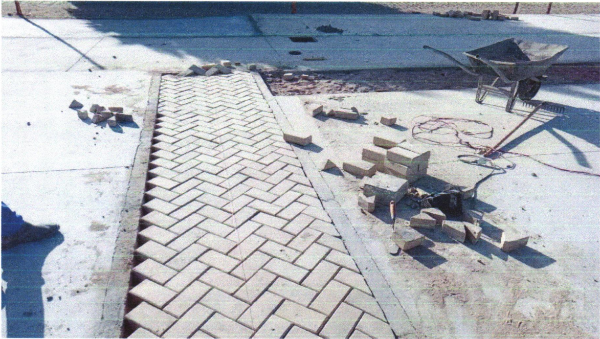
Foto 03 - Pavimentação em bloco de concreto vibroprensado, intertravado, colorido, 10x20cm, e=6cm, 46un/m 2 , NBR9781, Fck(min)=35MPa, sob coxim areia grossa compactada c/ placa vibratória, e(comp.)=6cm, rejuntado c/ areia fina.
